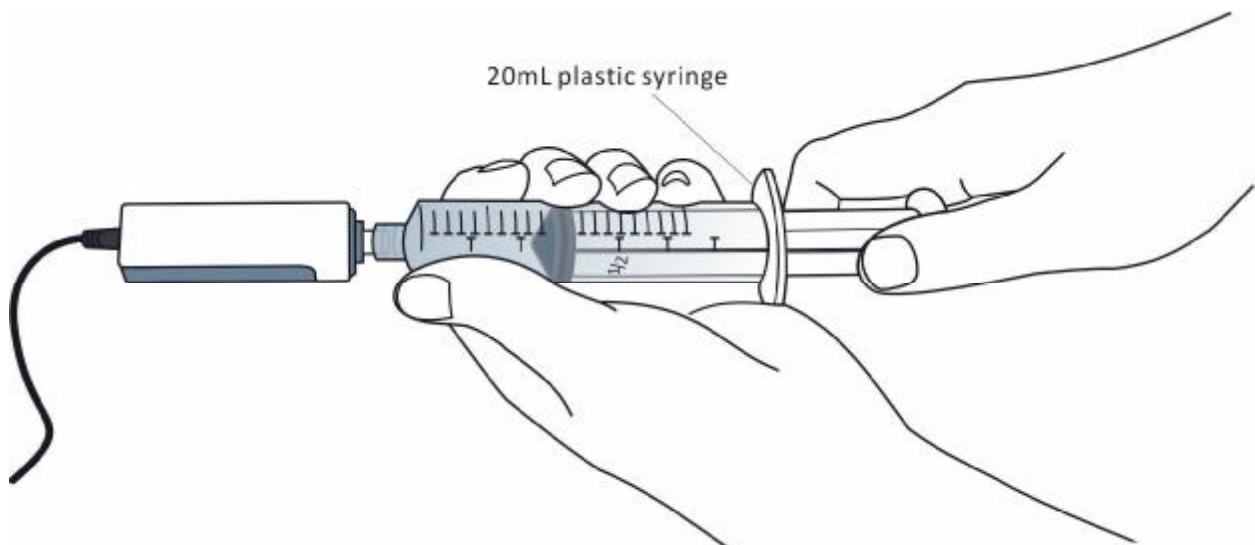
Obr. 1. Aparatúra na overenie Boylovho zákona.
